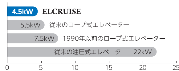
▲電動機容量の変遷(弊社) 乗用11人乗り速度60m/minの場合
